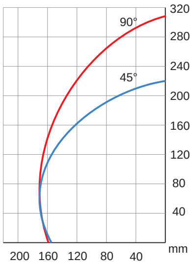
Sägeblatt Ø 500 mm Schnittdiagramm DGL 200E
